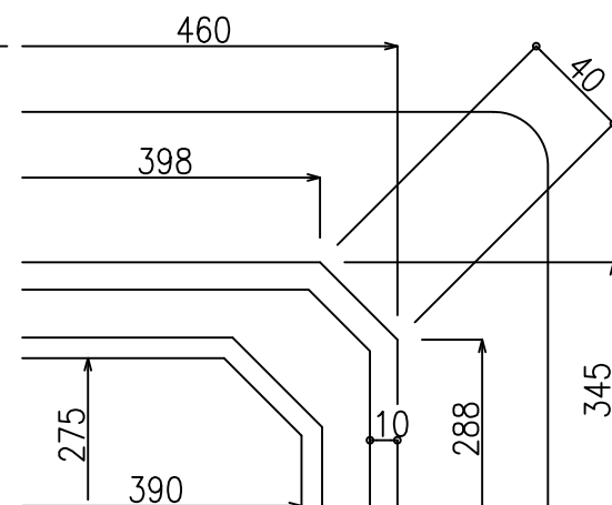
底ヨリノ詳細図
