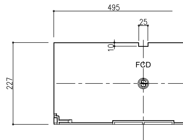
蓋裏面図
