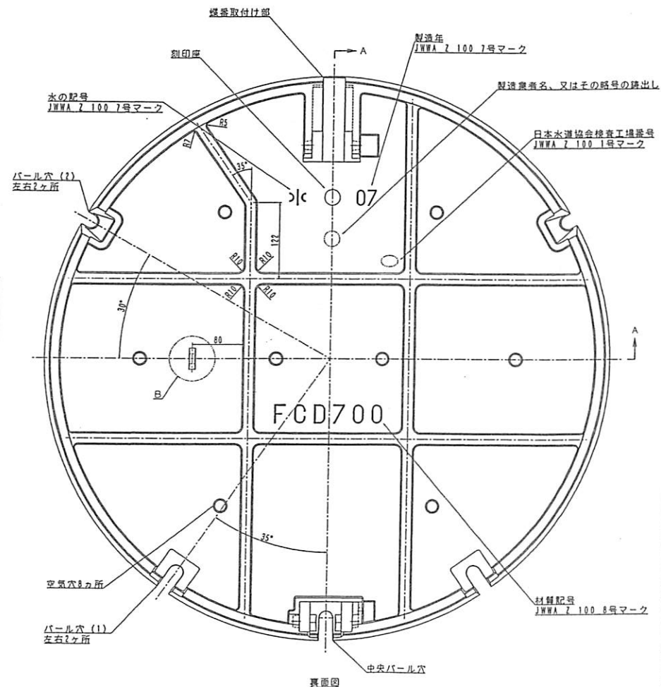
裏面図
