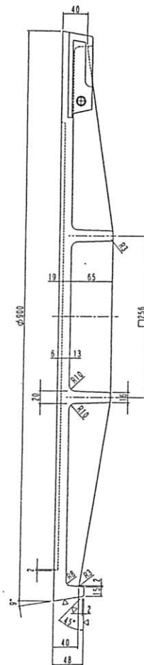
A-A断面図
