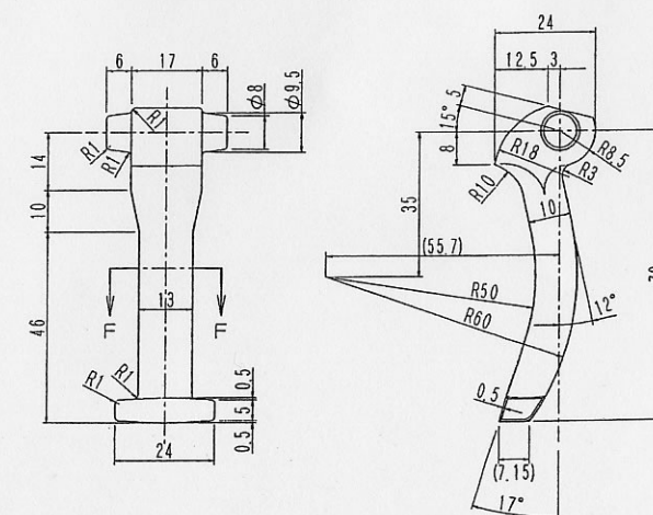
② 蝶番詳細図
