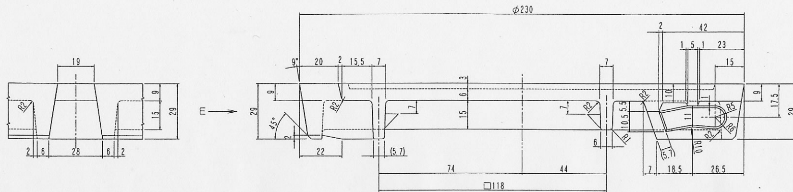
A—A 断面图
