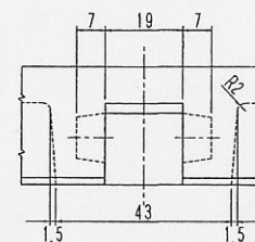
D 矢視図
