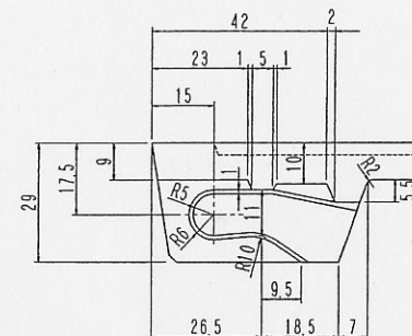
B-B 断面图
