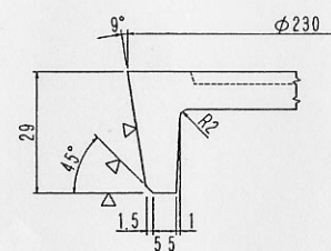
C - C 断面图
