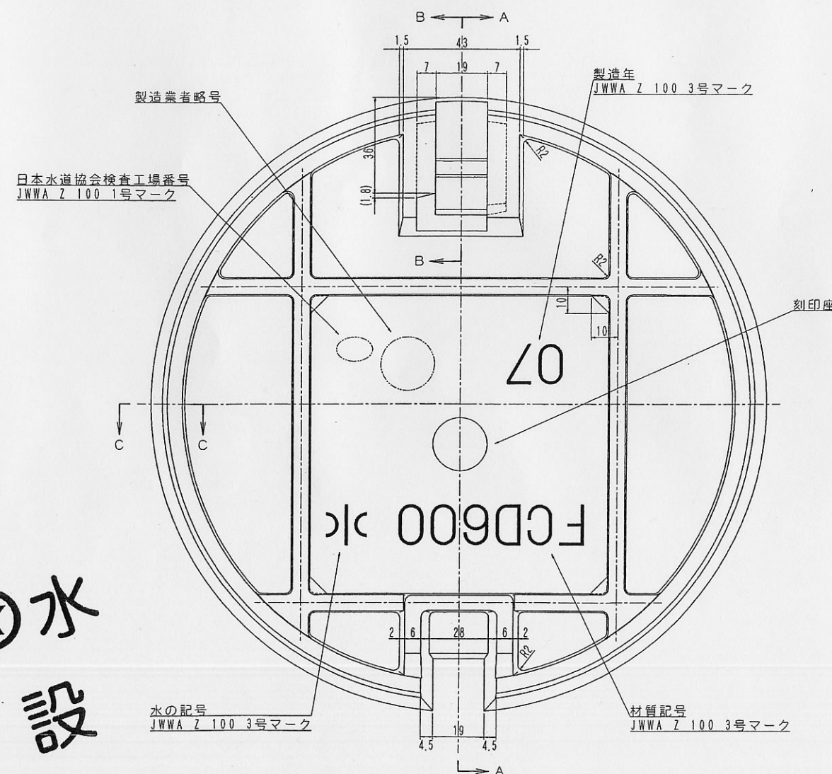
裏面図
