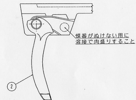
蝶番取付図
