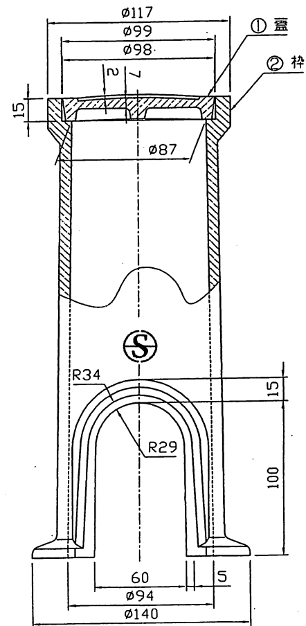
A-A矢視図
