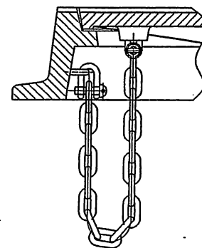
鎖取付部拡大図 ( Sc=1/4 )
